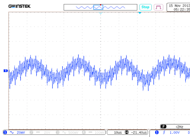
Рис. 22. Пульсации U_{\text{ВЫХ.НОМ}} .
