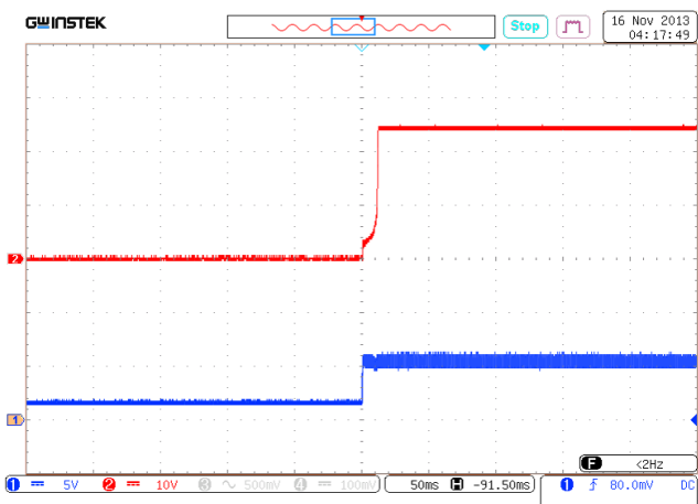
Рис. 20. Установление U_{\text{ВЫХ.НОМ}} с момента подачи ДУ (управляющий сигнал).
