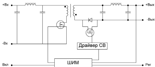
Рис. 1. Топология VDMC50.
