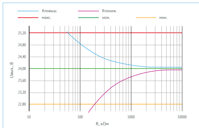
Рис. 9. График зависимости для U_{\text{вых.}}=24\text{ В} .
