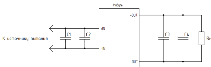
Рис. 2. Типовая схема включения VDMC50.
