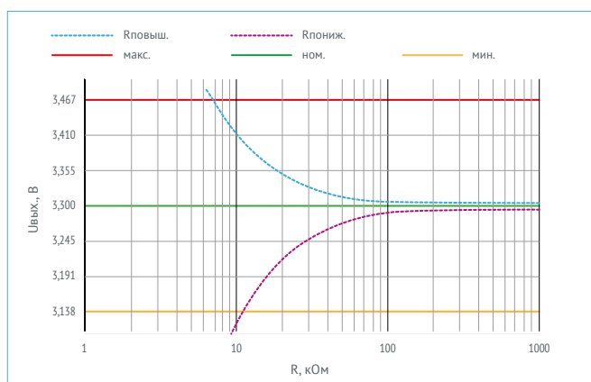
Рис. 4. График зависимости для U_{вых.}=3,3 В.
