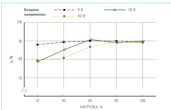
Рис. 14. VDMC50B12.
