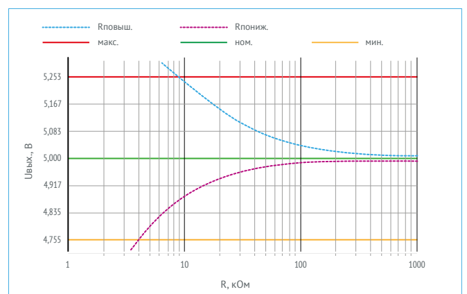
Рис. 5. График зависимости для U_{вых.}=5 В.
