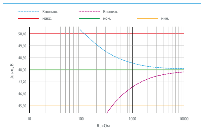
Рис. 11. График зависимости для U_{\text{вых.}}=48\text{ В} .
