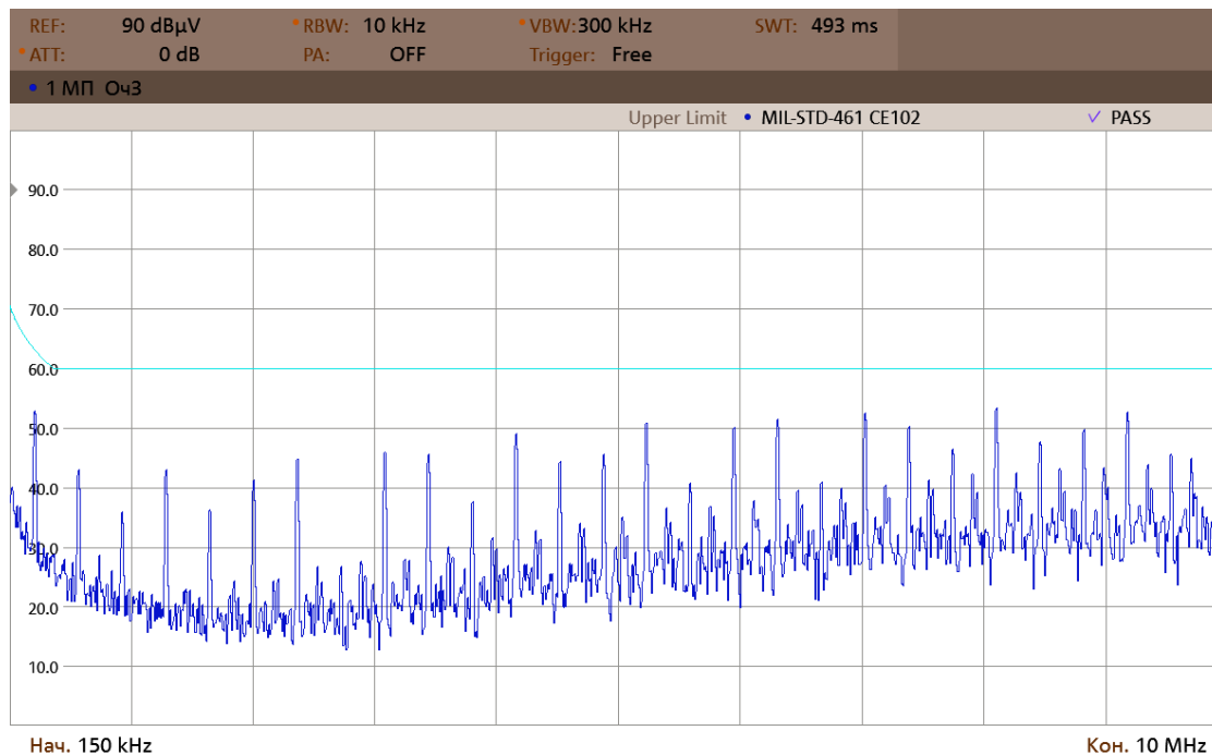
Рис. 24. Спектрограмма соответствия MIL-STD-461 (0,15-10 MHz).
