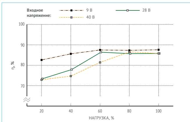
Рис. 18. VDMC50B48.
