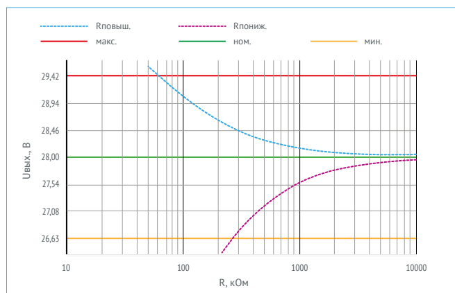
Рис. 10. График зависимости для U_{\text{вых.}}=28\text{ В} .
