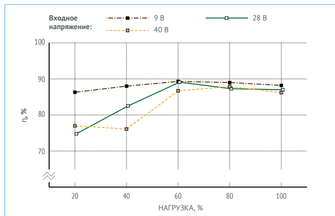
Рис. 15. VDMC50B15.
