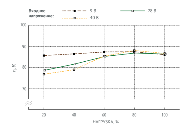
Рис. 17. VDMC50B28.
