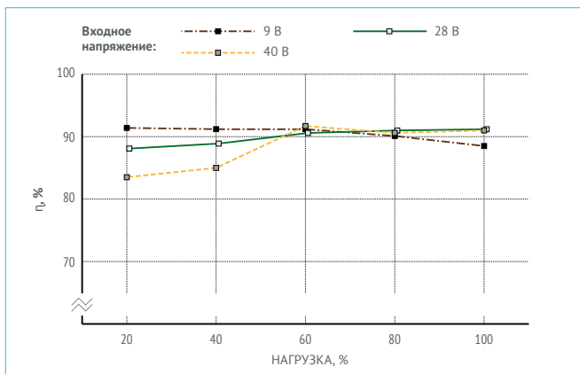
Рис. 12. VDMC50B05.
