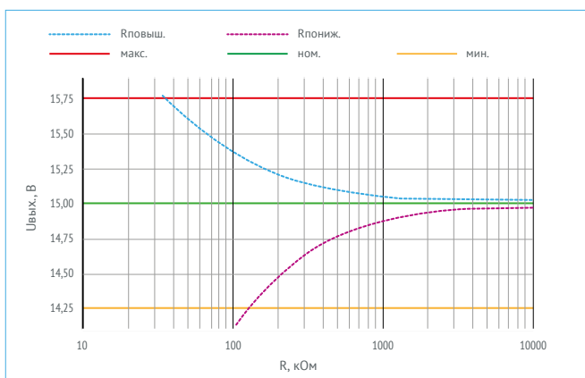
Рис. 8. График зависимости для U_{\text{вых.}}=15\text{ В} .
