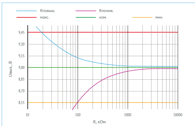
Рис. 6. График зависимости для U_{\text{вых.}}=9\text{ В} .
