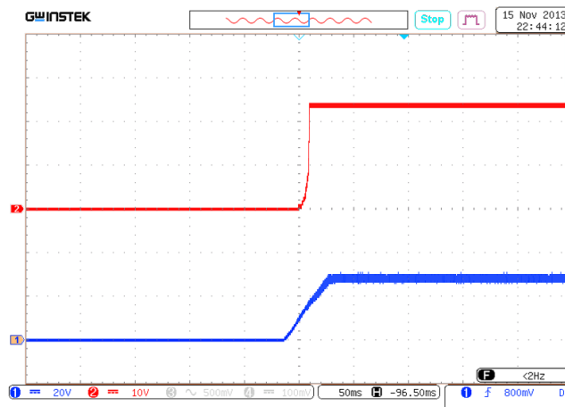
Рис. 21. Установление U_{\text{ВЫХ.НОМ}} с момента подачи U_{\text{ВХ.НОМ}} .
