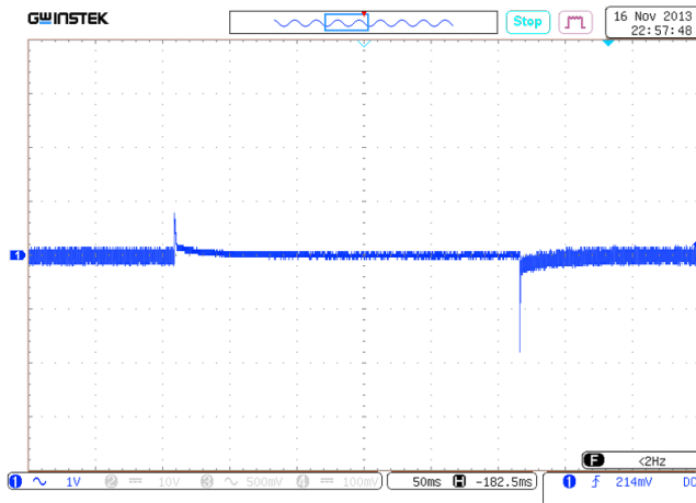
Рис. 23. Переходное отклонение выходного напряжения при изменении выходного тока от 75 до 100%.
