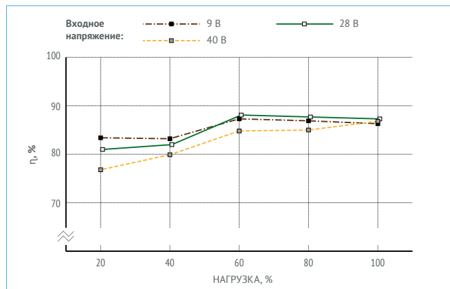
Рис. 16. VDMC50B24.
