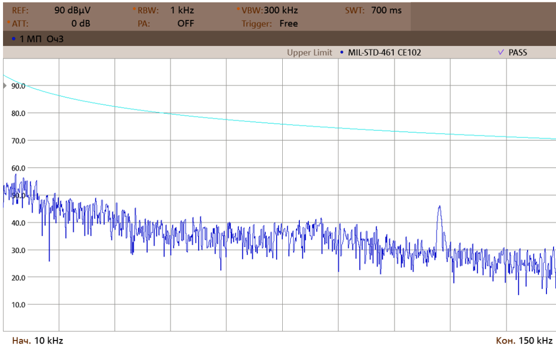
Рис. 25. Спектрограмма соответствия MIL-STD-461 (10–150 kHz).
