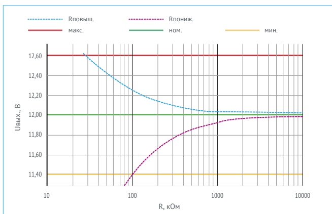
Рис. 7. График зависимости для U_{\text{вых.}}=12\text{ В} .
