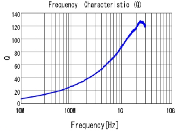
■ LQW18AN6N2C00 Q
