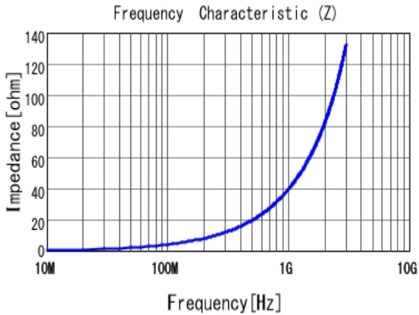
■ LQW18AN6N2C00 |Z|
