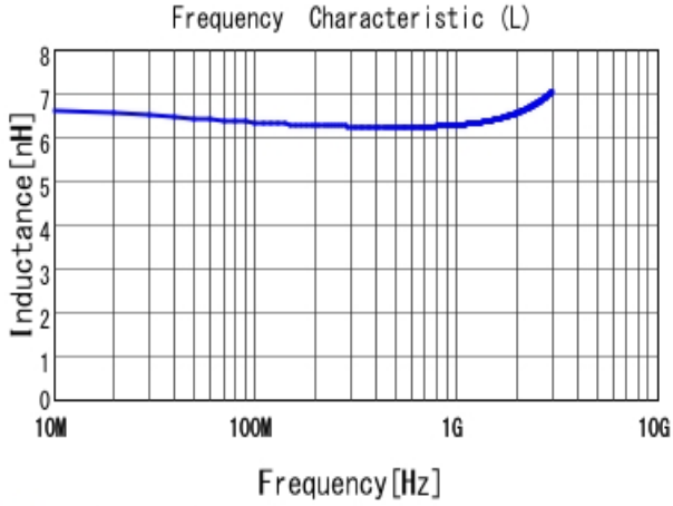
■ LQW18AN6N2C00 L
