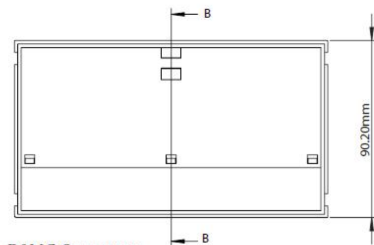
D9MG Основание
