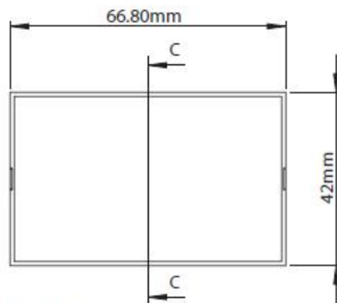
D4MG Крышка
