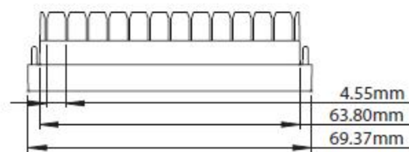
D4MG Заглушка
