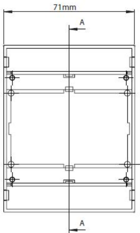
D4MG Корпус
