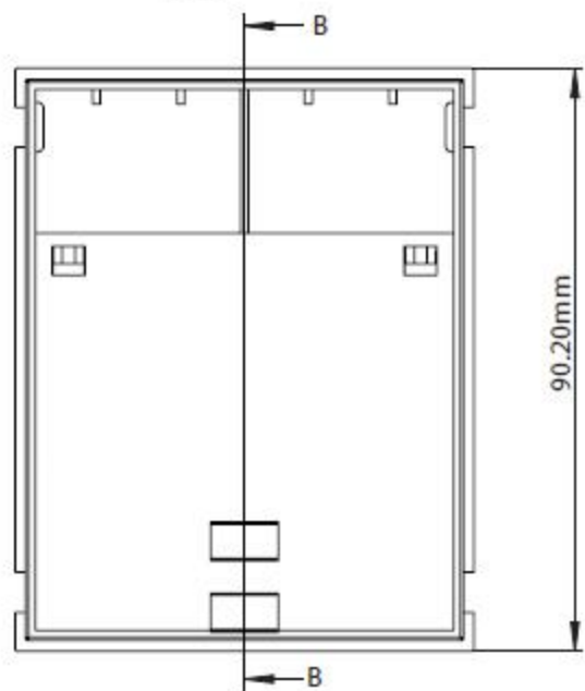
D4MG Основание
