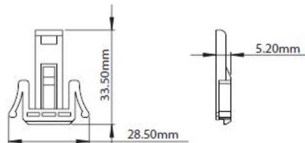
D3MG Крепеж на рейку
