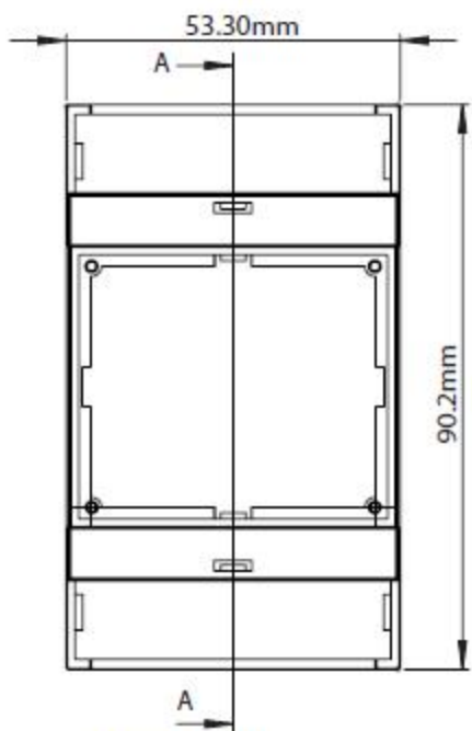
D3MG Корпус
