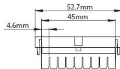
D3MG Заглушка
