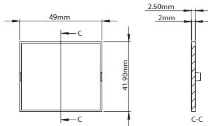
D3MG Крышка
