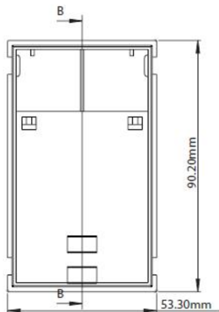
D3MG Основание
