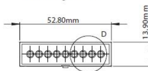
D3MG Крышка
