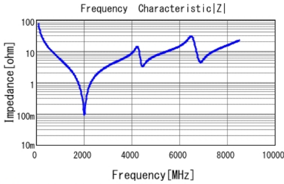
■ GCQ1555C1H220FB01 |Z| DC0V, 25degC
