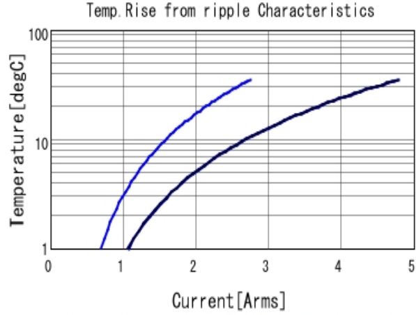
■ GCM21BR71C225KA64 Temp. rise ■ 100kHz ■ 500kHz ■ 1MHz
