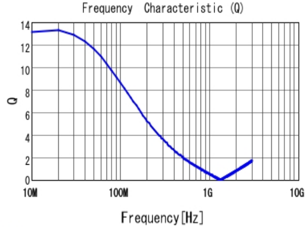
■ LQW18CNR27J00 Q
