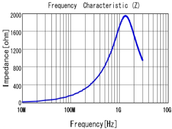
■ LQW18CNR27J00 |Z|
