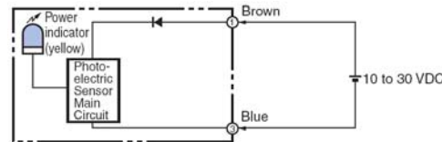
E3H2-T4 emitter
