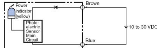
E3H2-T2 emitter
