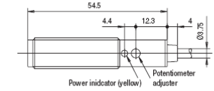
E3H2-T4 Emitter
