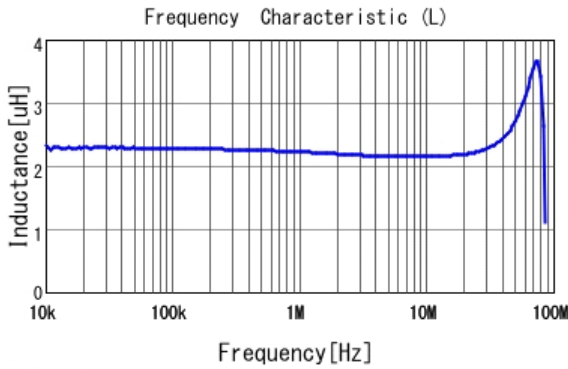
■ LQH2HPZ2R2MJR L
