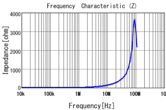
■ LQH2HPZ2R2MJR |Z|
