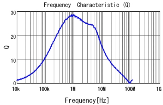
■ LQH2HPZ2R2MJR Q
