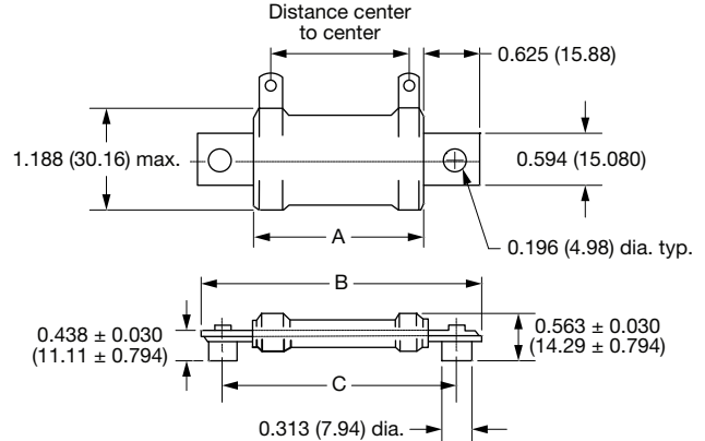
FSOT...XX FLAT 30 / 40 / 55 / 70 / 95
