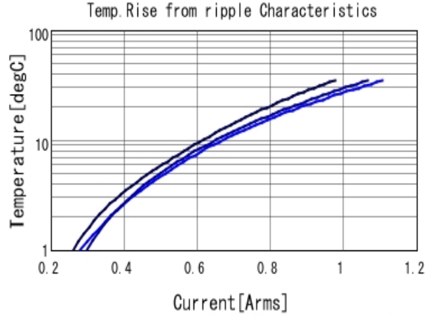
GJM1555C1H120JB01 Temp. rise 700MHz 1GHz 2GHz
