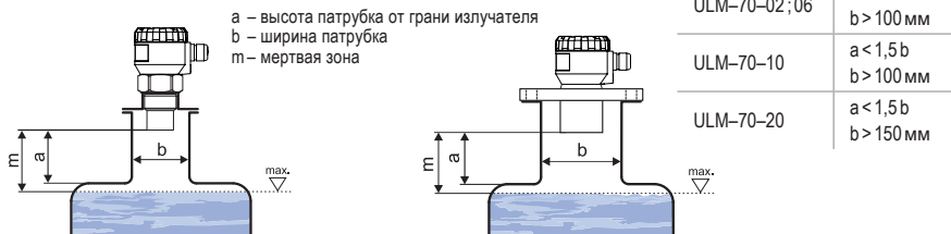
Рис. 4: Инсталляция измерителя уровня во входном патрубке
