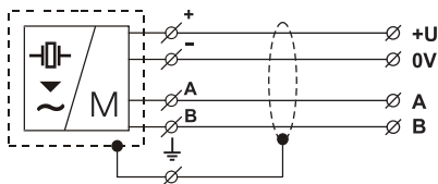
Рис. 21: Схема присоединения измерителя уровня с протоколом Modbus ULM-70_--M
