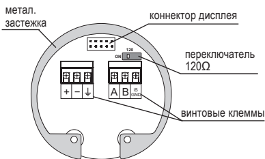
Рис. 22: Вид изнутри на винтовые клеммы измерителя уровня с протоколом Modbus ULM-70_--M
