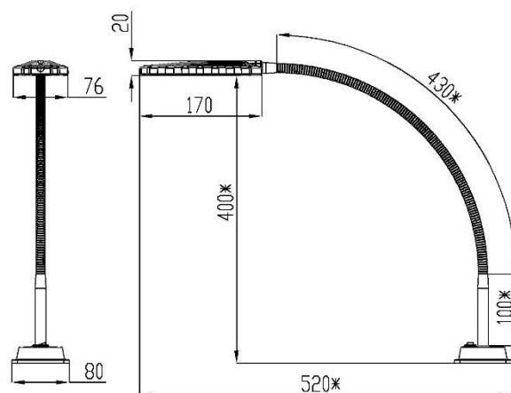
Рисунок – Внешний вид «Армата 045»
