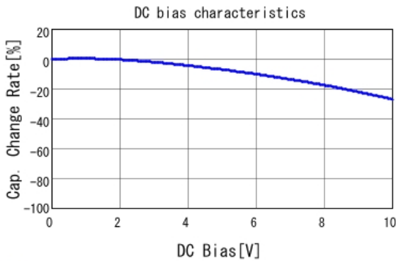
■ GRM188R71A684KA61 C-DC bias capchange, 25.0degC, AC1.
