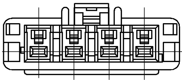
断面 A-A SECT A-A
