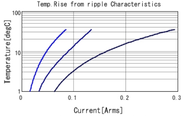
GCJ31BR73A472KXJ1 Temp. rise — 30kHz — 100kHz
