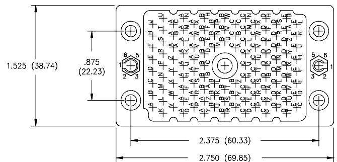
120 PIN RECEPTACLE
