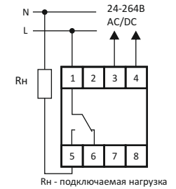
Rn - подключаемая нагрузка
