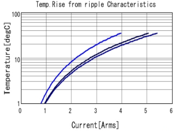
GRM31CR61A475KA01 Temp. rise ■ 100kHz ■ 500kHz ■ 1MHz
