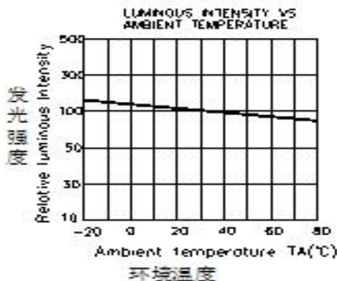
发光强度与环境温度关系
