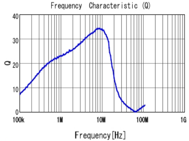
■ LQM31PN2R2M00 Q
