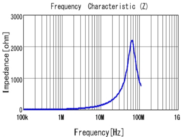
■ LQM31PN2R2M00 |Z|
