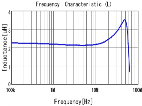
■ LQM31PN2R2M00 L
