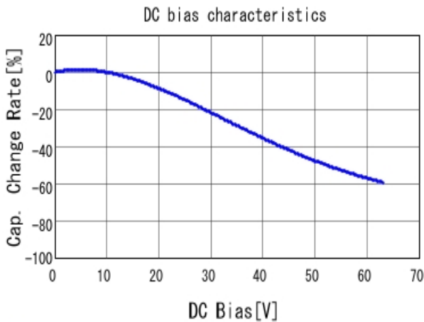
■ KRM55WR71J226MH01 C-DC bias capchange, 25.0degC, ACO.
