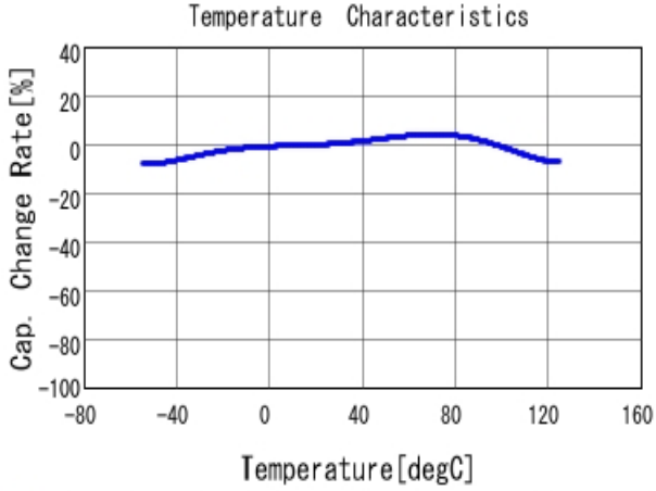
■ GRM31CR70J226ME19 C-Temp. capchange, DCO. 0V, ACO. 5V rm
