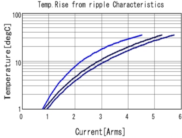
GRM31CR70J226ME19 Temp. rise ■ 100kHz ■ 500kHz ■ 1MHz
