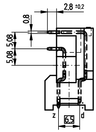
Bestückungsplan / contact layout
