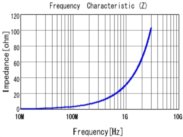
■ LQW15AN5N1D00 |Z|
