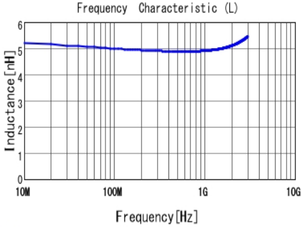
■ LQW15AN5N1D00 L
