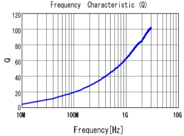
■ LQW15AN5N1D00 Q
