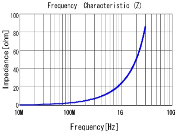
■ LQG15HS3N9S02 |Z|
