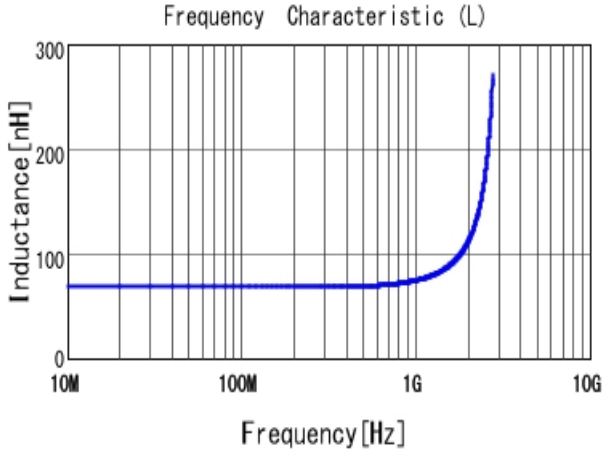
■ LQW15AN68NJ00 L
