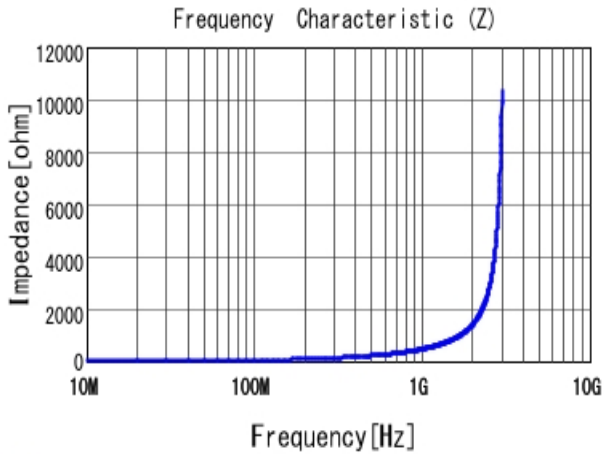
■ LQW15AN68NJ00 |Z|
