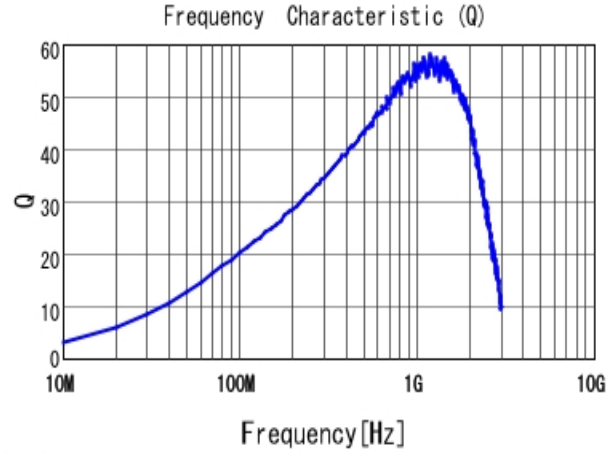
■ LQW15AN68NJ00 Q
