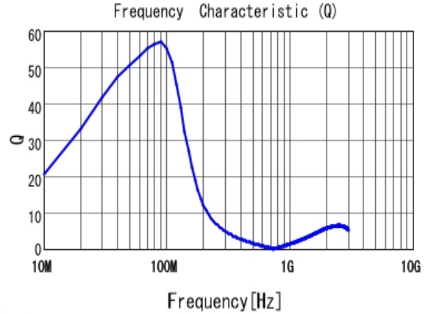
■ LQW21HNR47J00 Q
