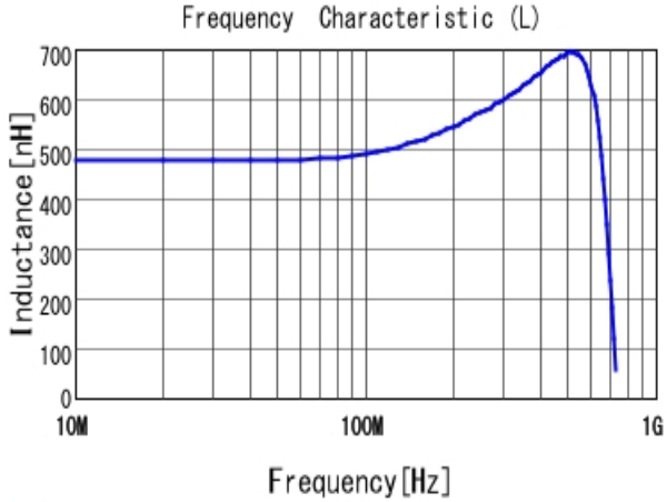
■ LQW21HNR47J00 L
