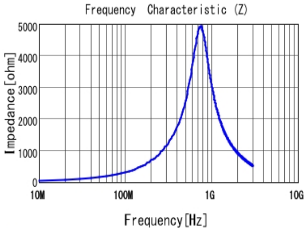
■ LQW21HNR47J00 |Z|
