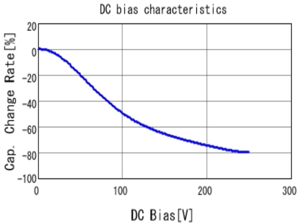
■ GCJ31BR72E223KXJ1 C-DC bias capchange, 25.0degC, AC1V
