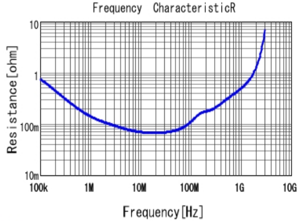
■ GCJ31BR72E223KXJ1 R DCOV, 25degC
