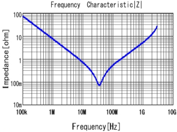
■ GCJ31BR72E223KXJ1 |Z| DCOV, 25degC
