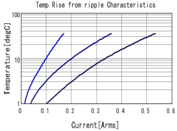
GCJ31BR72E223KXJ1 Temp. rise ■ 30kHz ■ 100kHz ■ 300kHz
