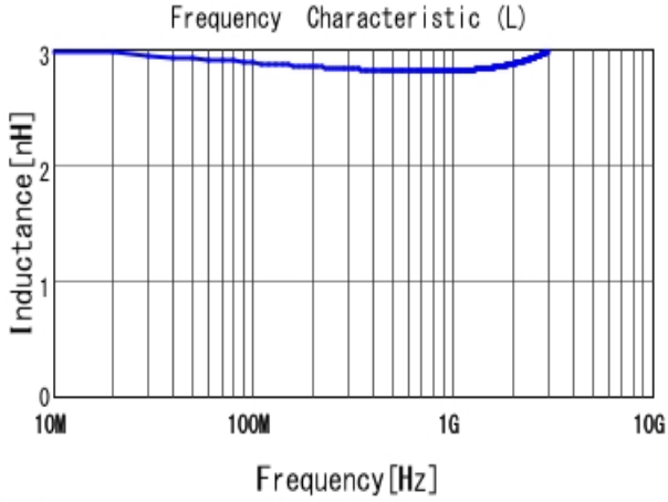
■ LQW15AN2N9C00 L
