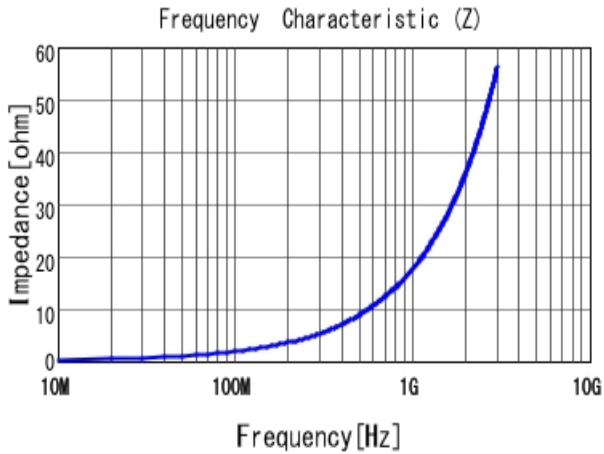
■ LQW15AN2N9C00 |Z|
