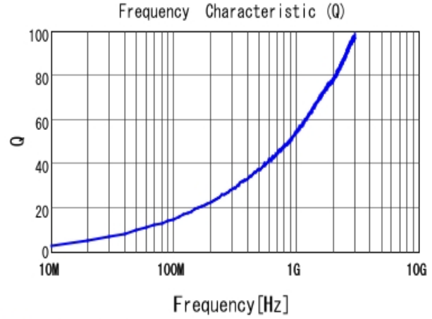
■ LQW15AN2N9C00 Q
