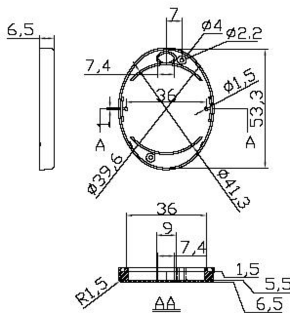
Bottom
