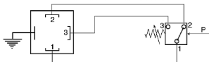
Connecteur électrique
