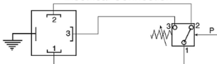
Elektrisches Anschlussbild
