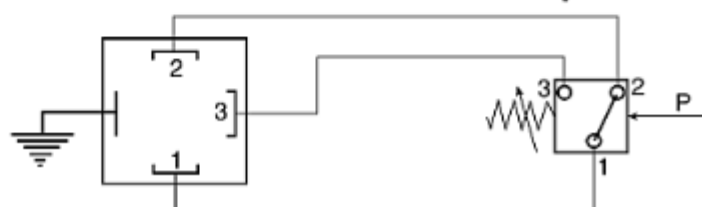
Connettori Elettronica
