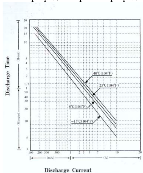
Ток разряда от времени разряда.
