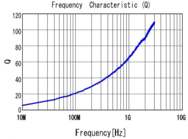
■ LQW15AN4N7C00 Q
