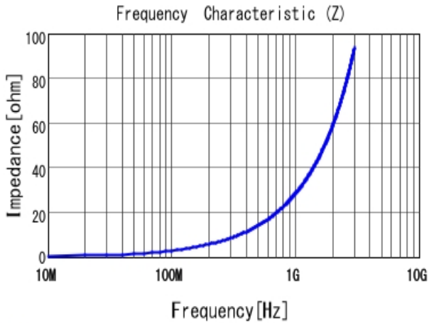
■ LQW15AN4N7C00 |Z|
