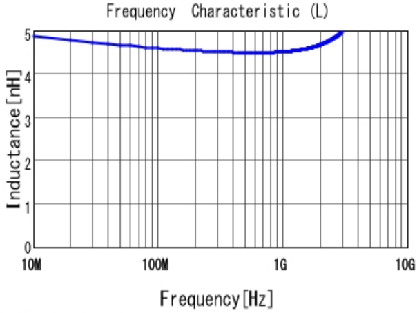
■ LQW15AN4N7C00 L
