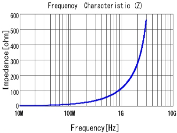
■ LQW18AN18NG00 |Z|
