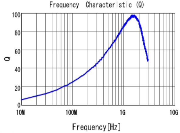
■ LQW18AN18NG00 Q
