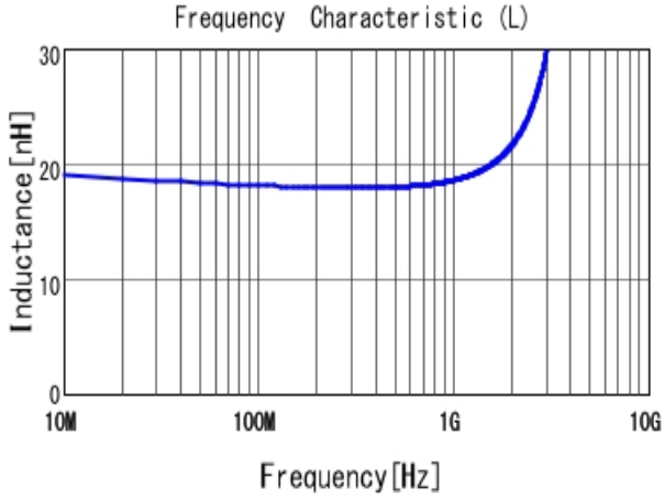
■ LQW18AN18NG00 L
