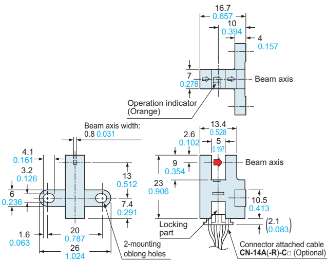
PM-T64W Sensor
