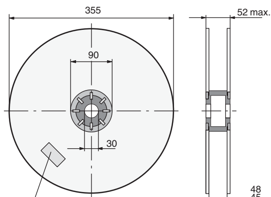
Fig. 20 - Reel
