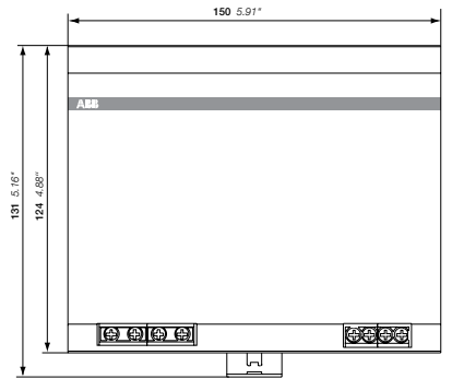
CP-T 24/20.0, CP-T 48/10.0
