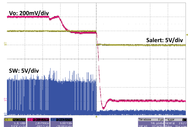
Fig. 34 - SiC451 UVP
