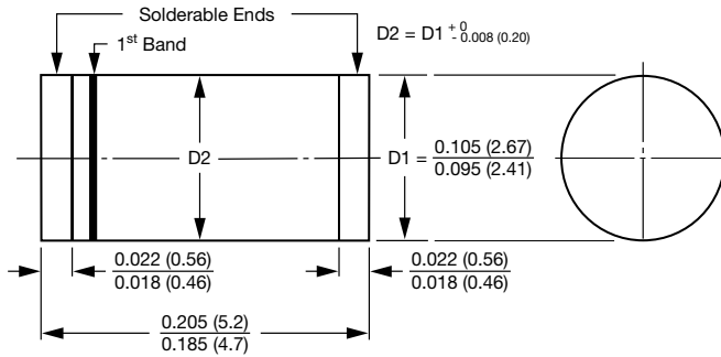
GL41 (DO-213AB)
