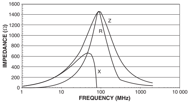
ILBB-0805 1500 \Omega
