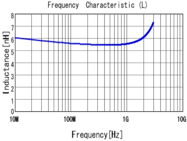
■ LQG18HN5N6S00 L
