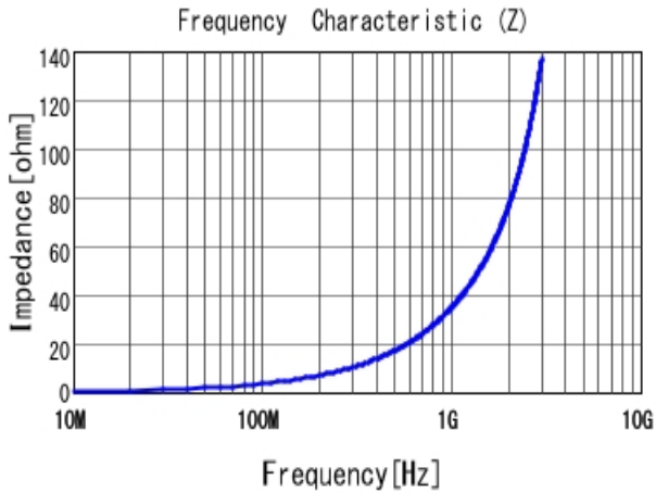
■ LQG18HN5N6S00 |Z|
