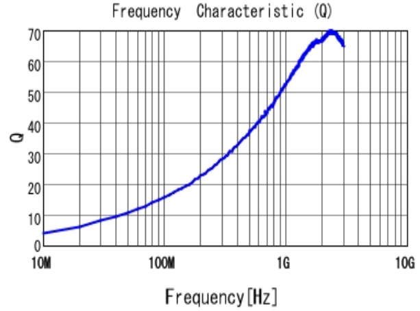
■ LQG18HN5N6S00 Q
