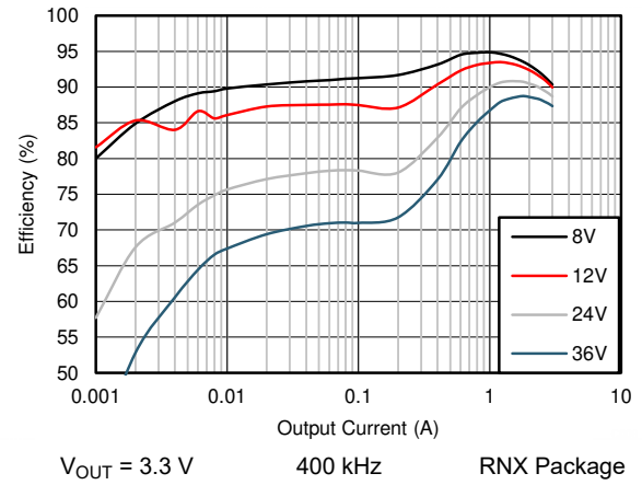
图 8-6. Efficiency
