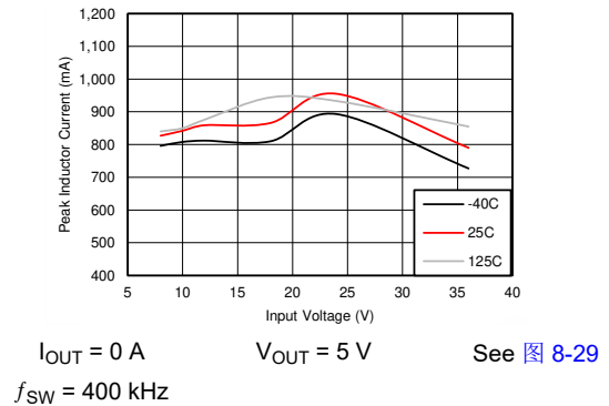
图 6-6. I_{PEAK-MIN}
