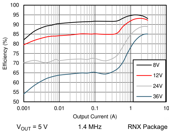
图 8-7. Efficiency
