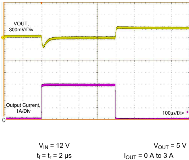
图 8-15. Load Transient
