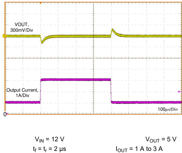
图 8-16. Load Transient
