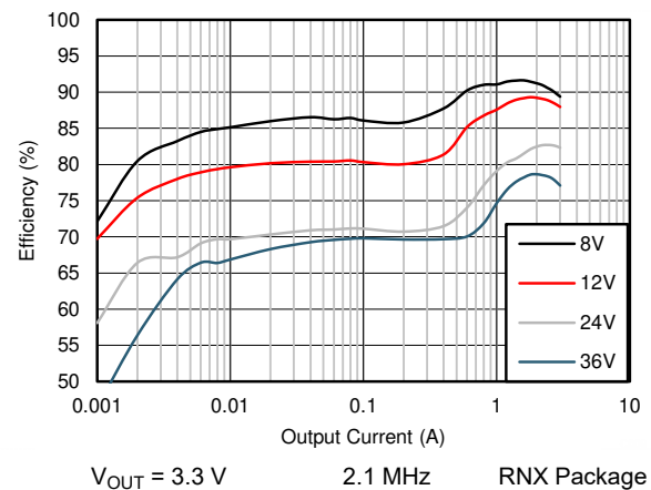
图 8-10. Efficiency
