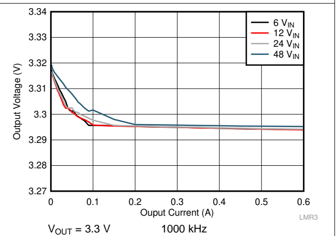
图 24. Load Regulation
