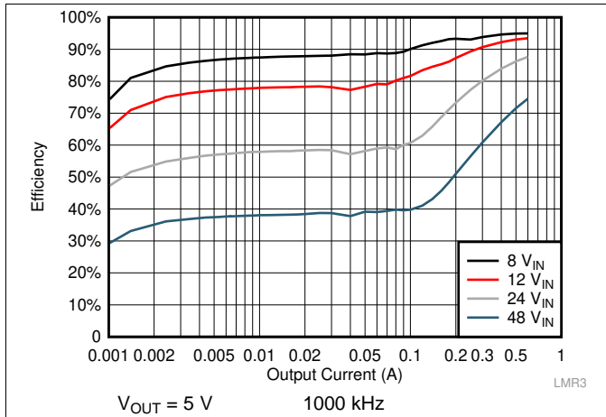
图 21. Efficiency
