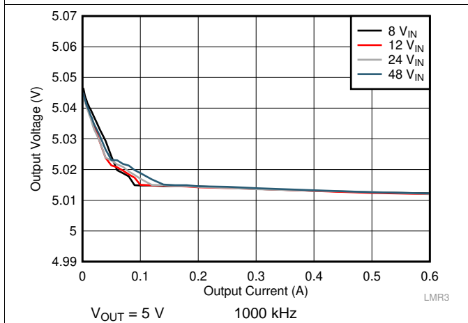
图 23. Load Regulation
