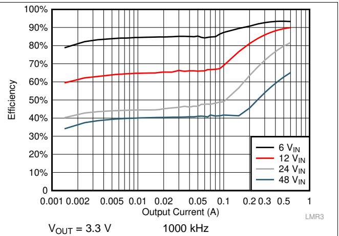
图 22. Efficiency
