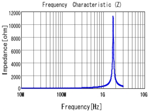
■ LQG15HN39NJ02 |Z|
