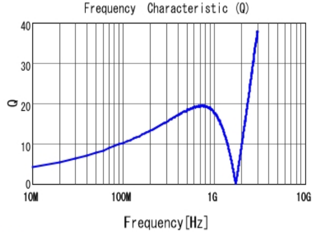
■ LQG15HN39NJ02 Q
