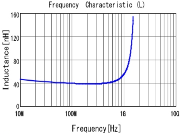
■ LQG15HN39NJ02 L
