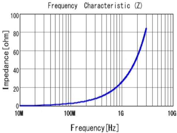
■ LQW15AN4N3D00 |Z|
