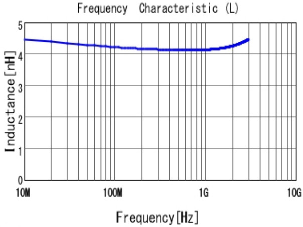
■ LQW15AN4N3D00 L
