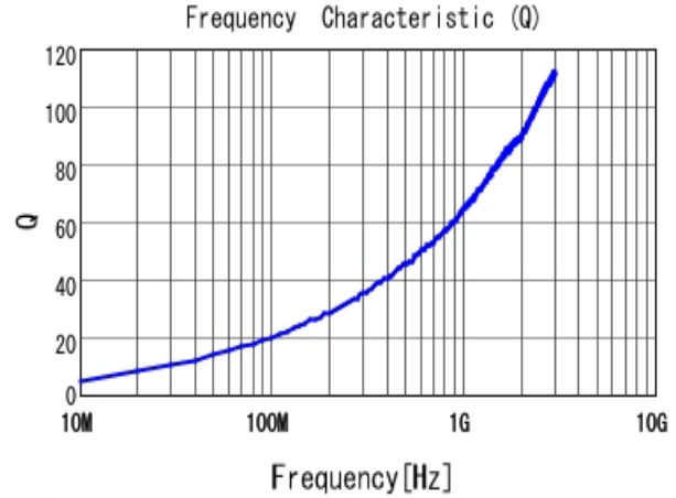
■ LQW15AN4N3D00 Q
