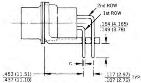
DE, DA, DB, DC SIZES
