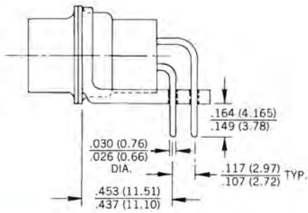
DE, DA, DB, DC SIZES
