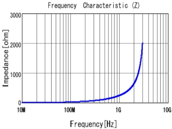
■ LQW18AN36NG00 |Z|
