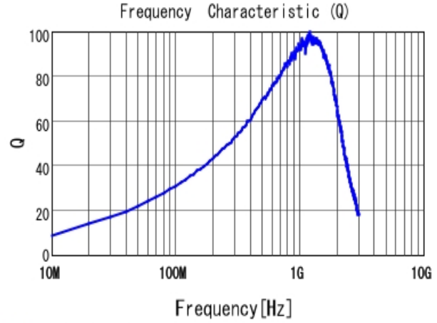
■ LQW18AN36NG00 Q
