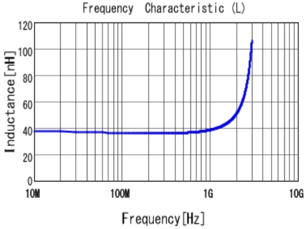
■ LQW18AN36NG00 L
