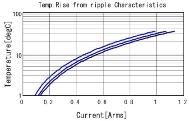
■ GRT033C81E104KE01 Temp. rise ■ 400kHz ■ 800kHz ■ 1MHz
