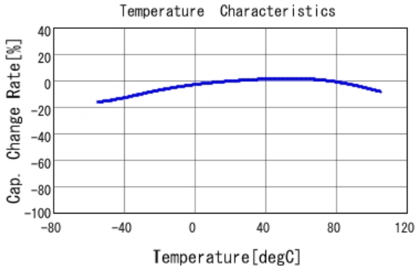
■ GRT033C81E104KE01 C-Temp. capchange, DCO. 0V, ACO. 2Vrm
